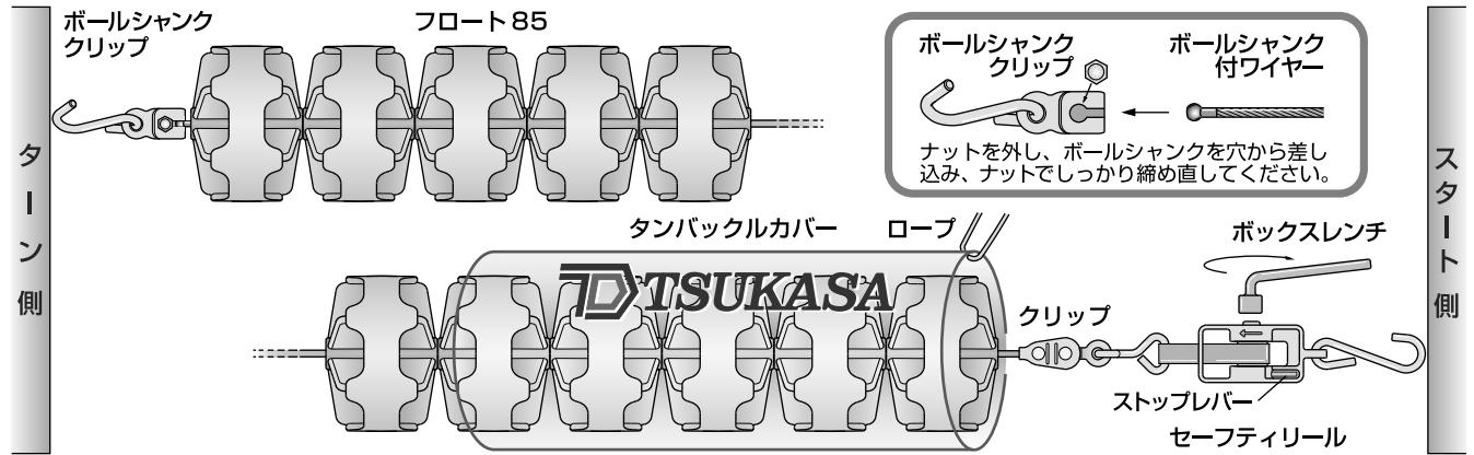
配列図
